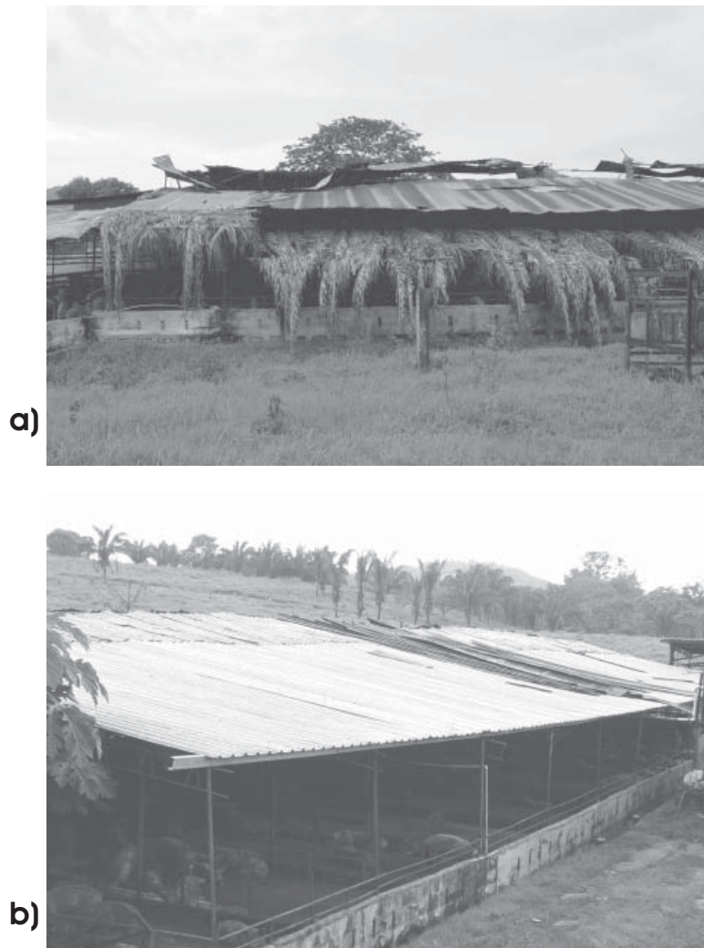
Figura 7.31. Estado de los techos: a) antes de P+L; b) después de P+L.
